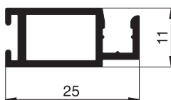
Bestell Nr.: 10 23 06 Bez.: Spannrahmenprofil
