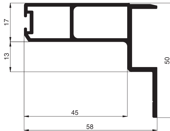
Bestell Nr.: 10 32 16 Bez.: Lichtschachtdeckungsprofil
