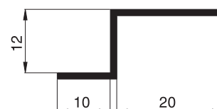
Bestell Nr.: 10 26 07 Bez.: Z-Schiene
