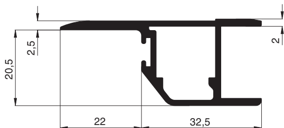
Bestell Nr.: 10 62 04 Bez.: Lichtschachtabdeckungsprofil
