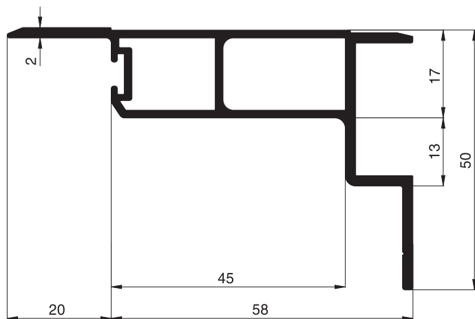
Bestell Nr.: 10 32 14 Bez.: Lichtschachtdeckungsprofil
