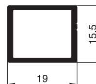
Bestell Nr.: 10 35 22 Bez.: Montagerahmenprofil
