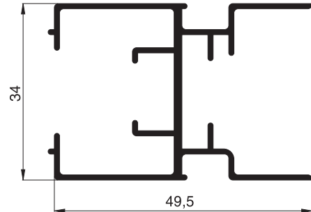
Bestell Nr.: 10 42 05 Bez.: bewegliches Flügelprofil
